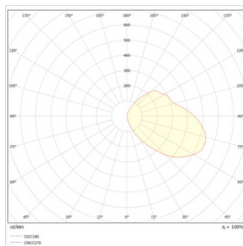
DPR20 AL Lichtverteilungskurve
