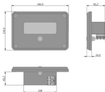
DPR20 AL Zeichnung
