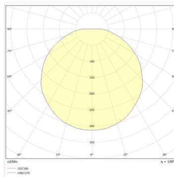
Torino G2 Lichtverteilungskurve
